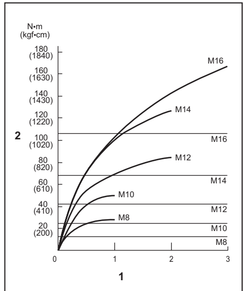
1. Kinnitamisaja (sekund) 2. Väändmoment
