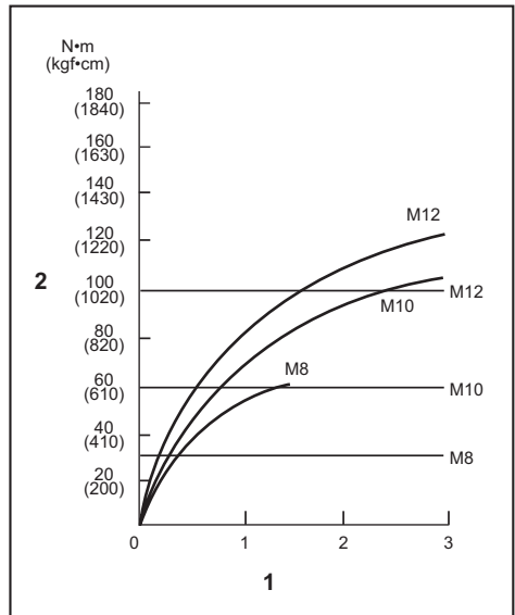
1. Festetid (sekunder) 2. Tiltrekingsmoment
